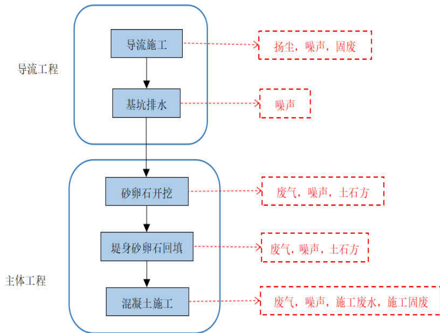
图 2-2 施工期堤防工程工艺流程及产污位置图
