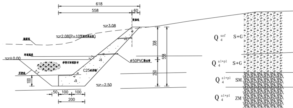
图 2-1 C25 砼仰斜式挡墙堤型
