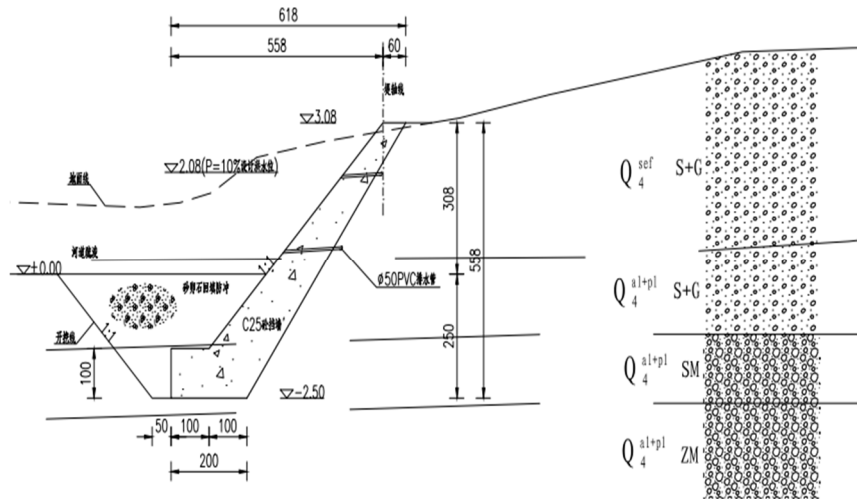
方案一：C25 砼仰斜式挡墙
