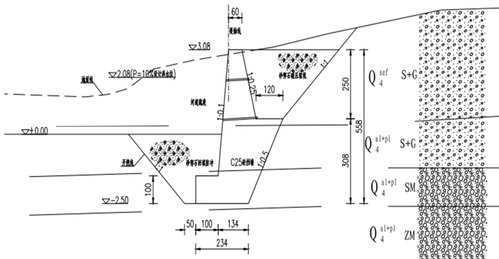
方案二：C25 砼衡重式挡墙
