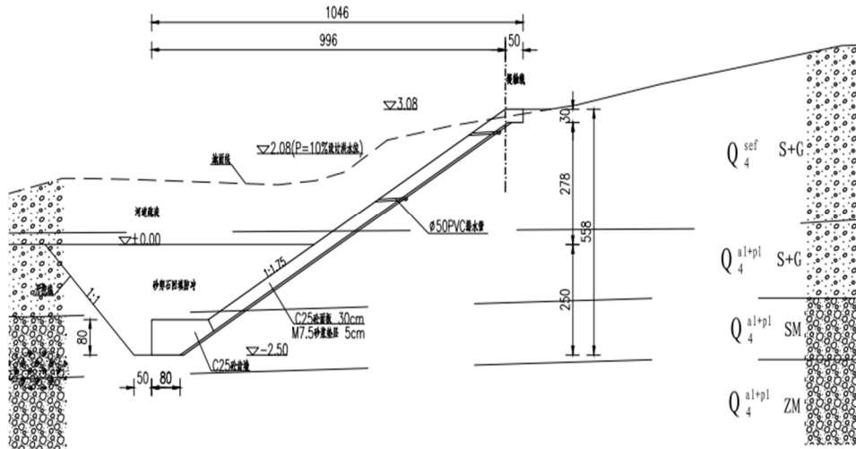
方案三：C25 砼斜坡式面板堤
